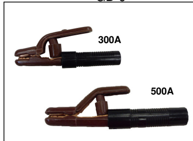
GD-J
