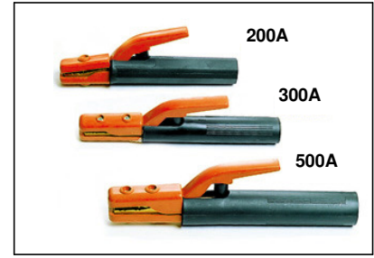
GD354A
